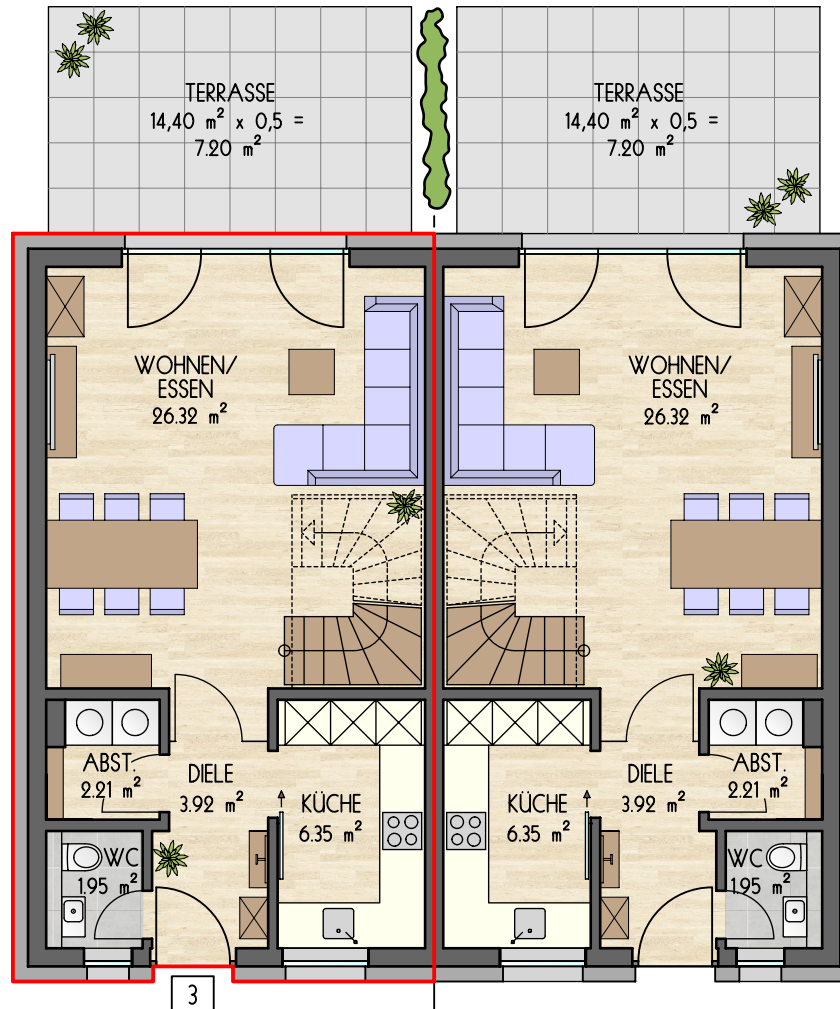
GRUNDRISS ERDGESCHOSS WOHNUNG 3
