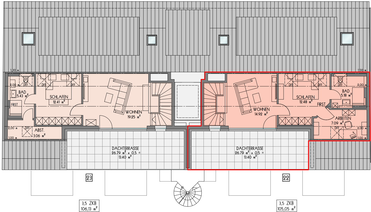
LAGE DER WOHNUNG IM GESCHOSS -OBERE EBENE- M 1:150
