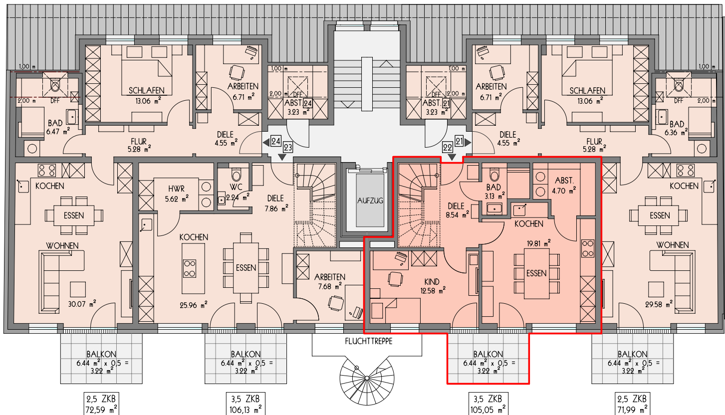
LAGE DER WOHNUNG IM GESCHOSS -UNTERE EBENE- M 1:150
