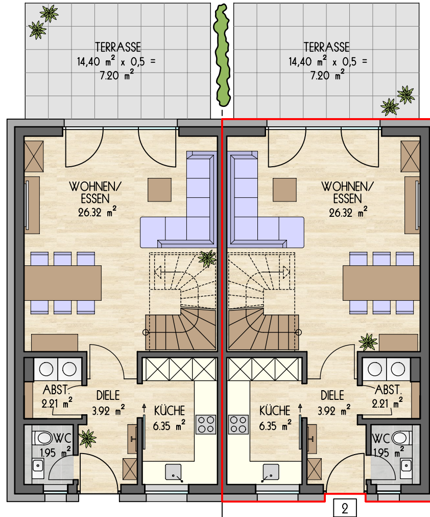
GRUNDRISS ERDGESCHOSS WOHNUNG 2
