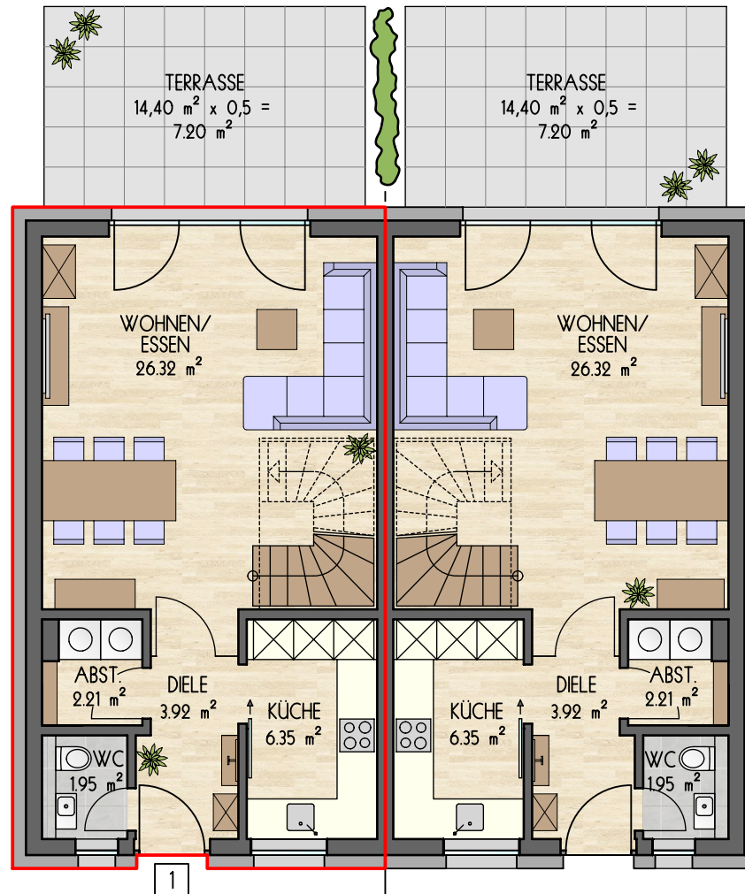
GRUNDRISS ERDGESCHOSS WOHNUNG 1
